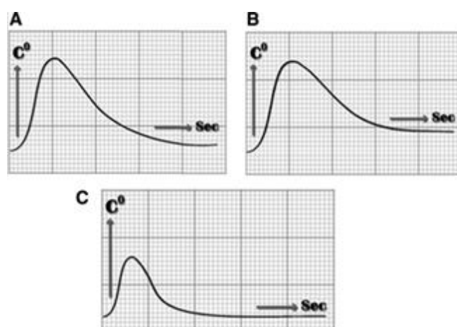
Рисунок 1.1 - Кривая термодилуции (А – норма - резкий начальный ход вверх, за которым следует возвращение к базовой линии; В - кривая низкого СВ, которая требует больше времени для достижения базовой линии и имеет большую площадь под кривой по сравнению с нормой; С - высокий СВ с его небольшой кривой и, соответственно, меньшей площадью под кривой) [35]
