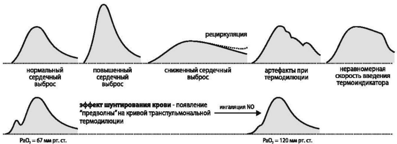
Рисунок 2.14 - Изменения формы кривой дилуции термоиндикатора [12]
