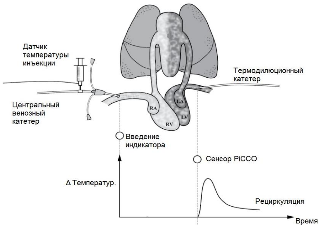
Рисунок 2.12 - Методика транспульмональной термодилуции [137]
