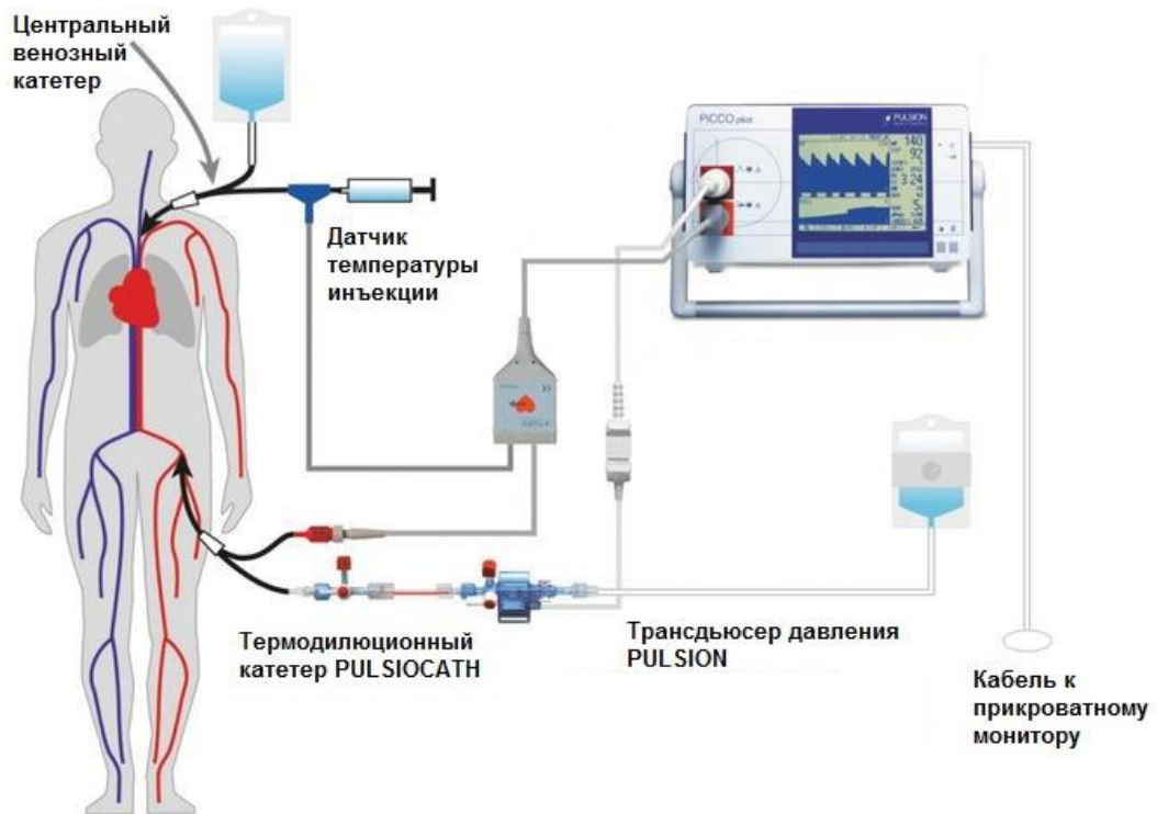
Рисунок 2.13 - Схематическое изображение системы PiCCO [135]
